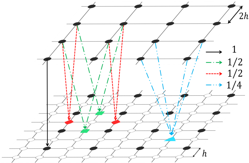
Figura 3.6: Prolongação utilizando interpolação bilinear.
