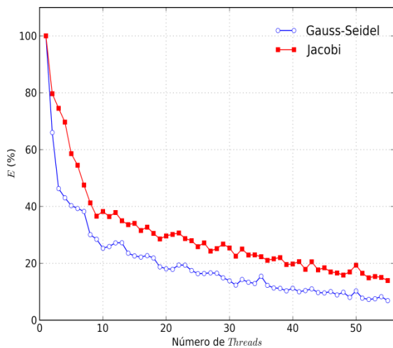
a) Eficiência para N = 513 \times 513
