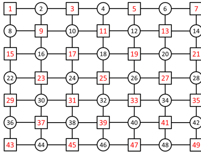
Figura 5.9: Ordenação da malha para Gauss-Seidel red-black .
