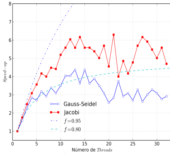
a) Speed-up para N = 129 \times 129
