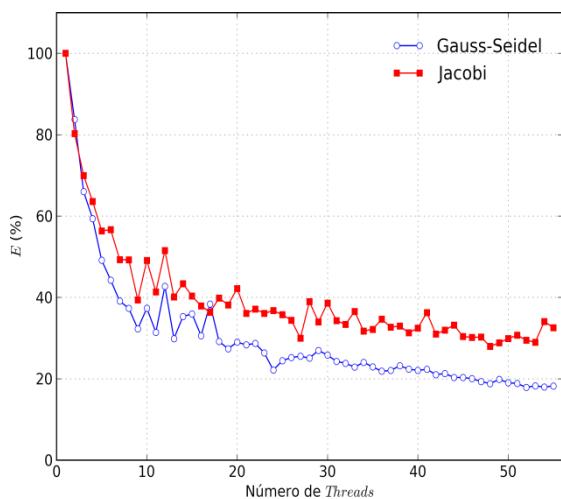
c) Eficiência para N = 2049 \times 2049
