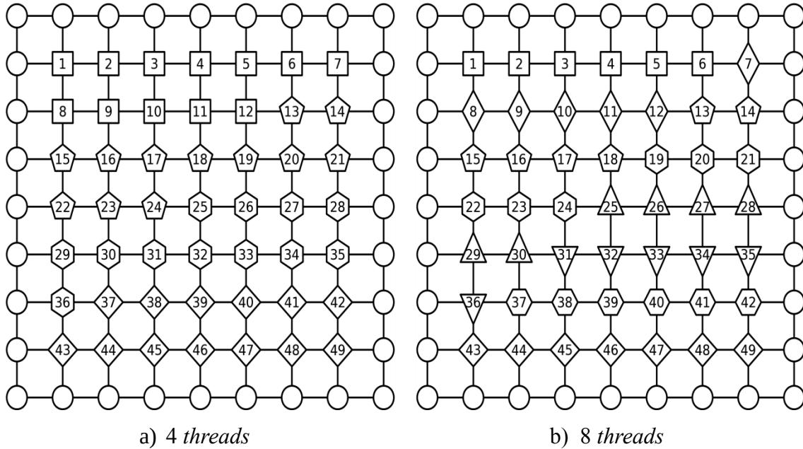
Figura 5.6: Domínio com 49 nós particionado em (a) 4 subdomínios e (b) 8 subdomínios.
