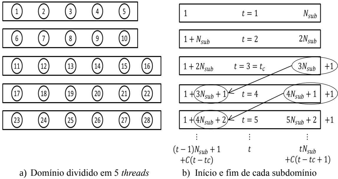
Figura 5.5: Divisão não exata de um subdomínio.
