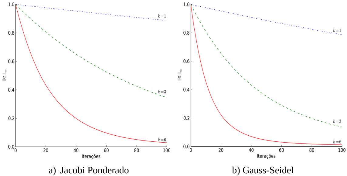
Figura 2.4: Norma infinito do erro numérico versus iterações para os métodos de Jacobi ponderado com \omega = 2/3 e Gauss-Seidel.
