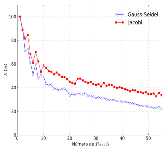
e) Eficiência para N = 8193 \times 8193
