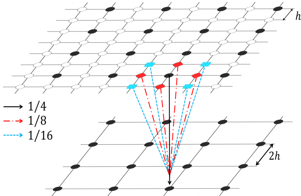
Figura 3.5: Restrição utilizando o operador de restrição por ponderação completa.
