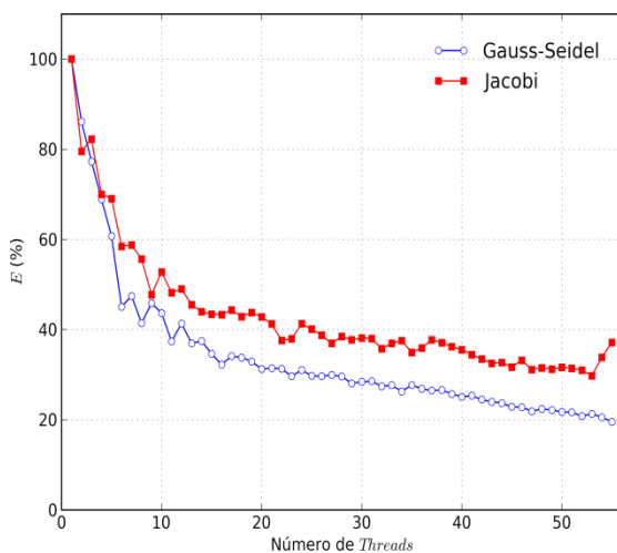
d) Eficiência para N = 4097 \times 4097
