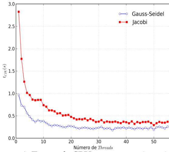
a) Tempo de CPU para N = 513 \times 513
