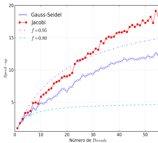
e) Speed-up para N = 8193 \times 8193
