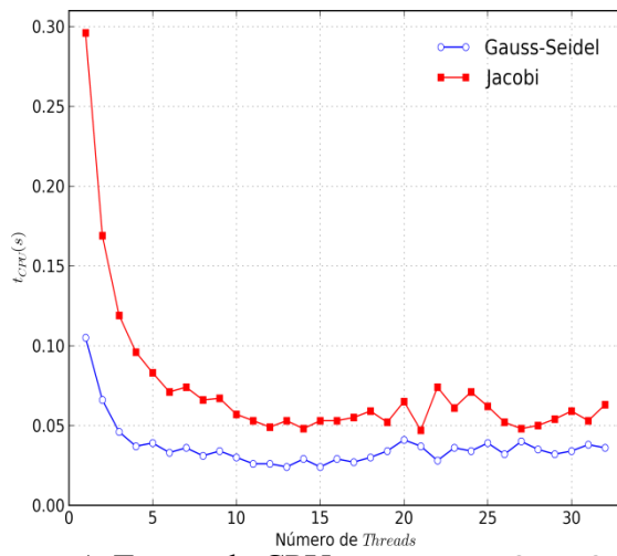
c) Tempo de CPU para N = 129 \times 129
