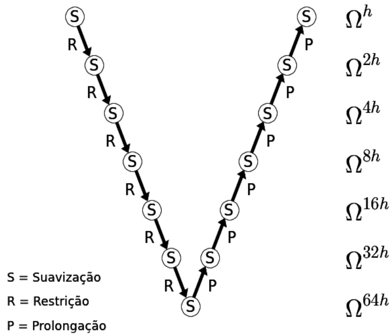
Figura 3.7: Diagrama do ciclo V.
