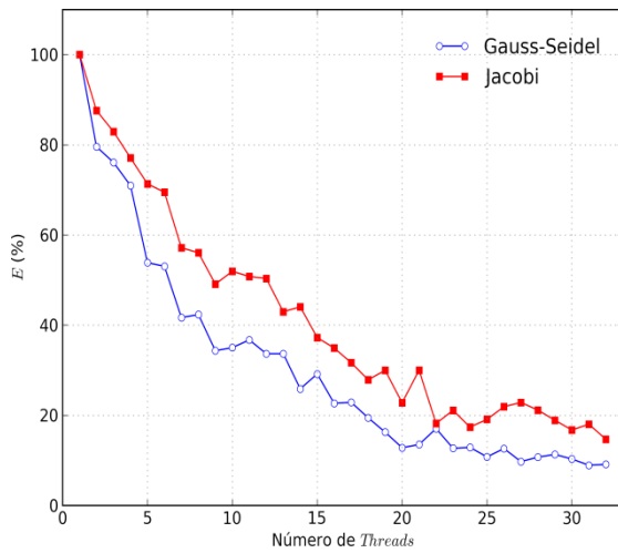
e) Eficiência para N = 129 \times 129
