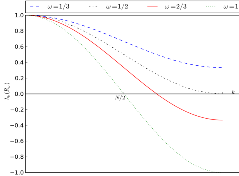
Figura 2.3: Autovalores da matriz de iteração R_\omega .
