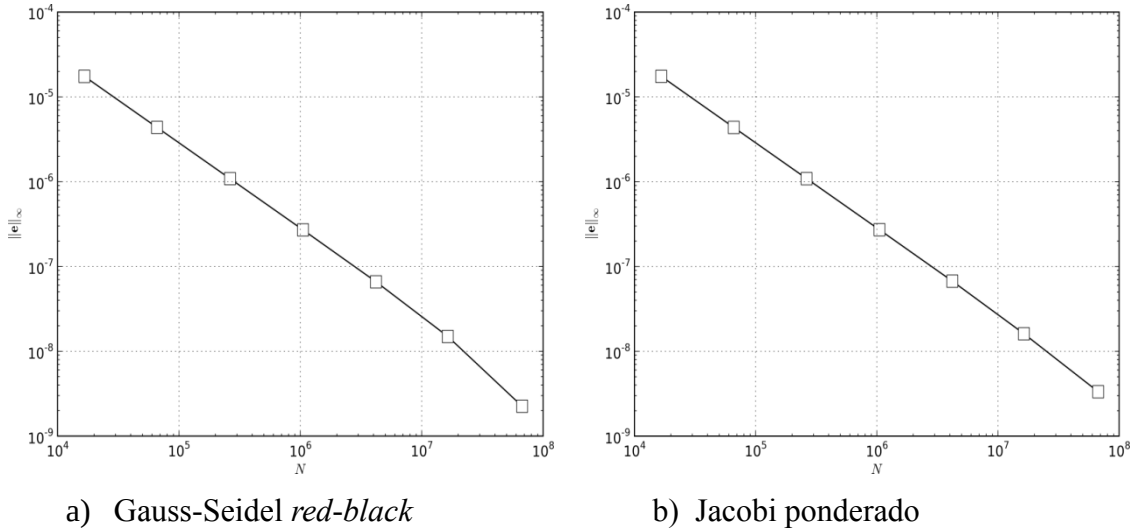
Figura 6.1: Norma infinito do erro numérico para o método multigrid utilizando os métodos Gauss-Seidel red-black e Jacobi ponderado.
