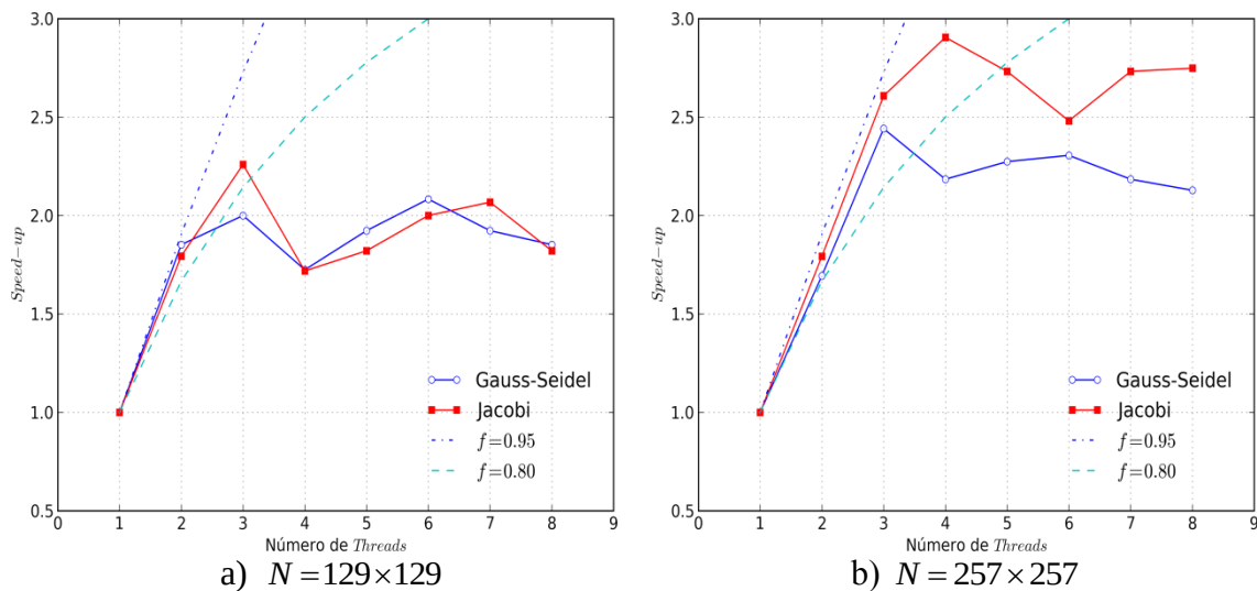
Figura A 1 : Speed-up oscilatório para Core I7
