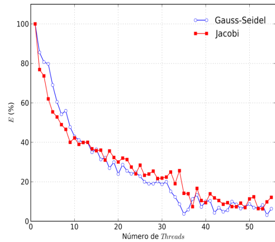
f) Eficiência para N = 257 \times 257
