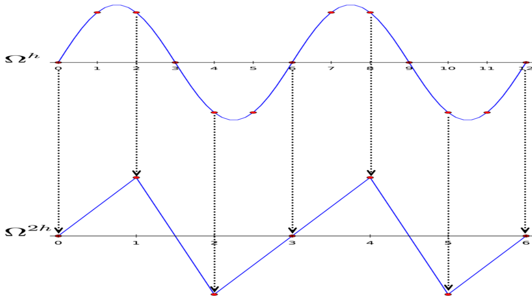
Figura 3.1: Número de ondas k = 4 sobre uma malha fina \Omega^h com N = 12 e sobre a malha imediatamente mais grossa \Omega^{2h} com N = 6 (BRIGGS et al, 2000).
