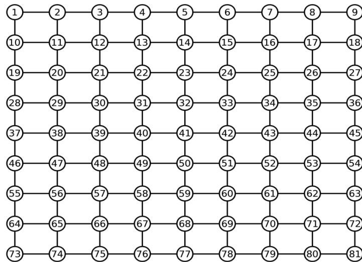
Figura 1.2: Ordenação lexicográfica.
