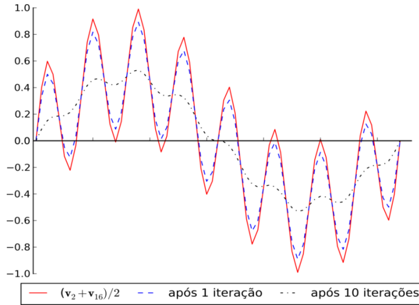
Figura 2.6: Método de Jacobi ponderado com \omega = 2/3 aplicado na estimativa inicial (v_2 + v_{16})/2 ao longo de 1 iteração e após 10 iterações (BRIGGS et al., 2000).
