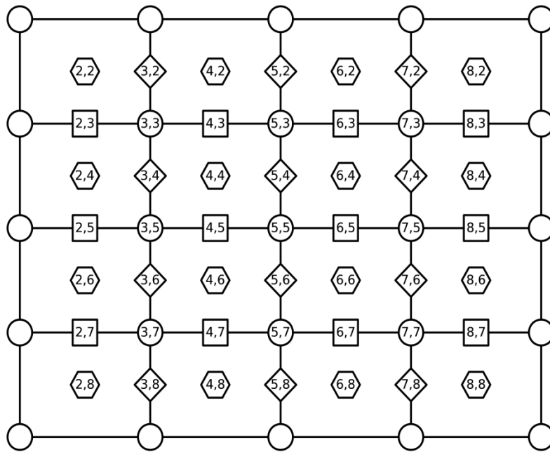
Figura 5.11: Malha fina sobreposta a uma malha grossa para razão de engrossamento r = 2 .
