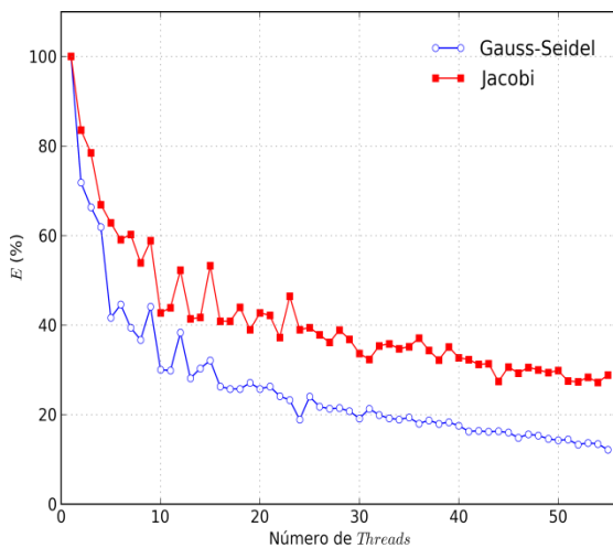
b) Eficiência para N = 1025 \times 1025
