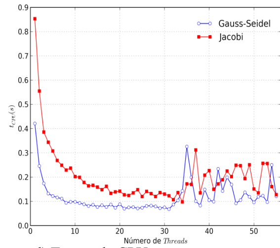
d) Tempo de CPU para N = 257 \times 257
