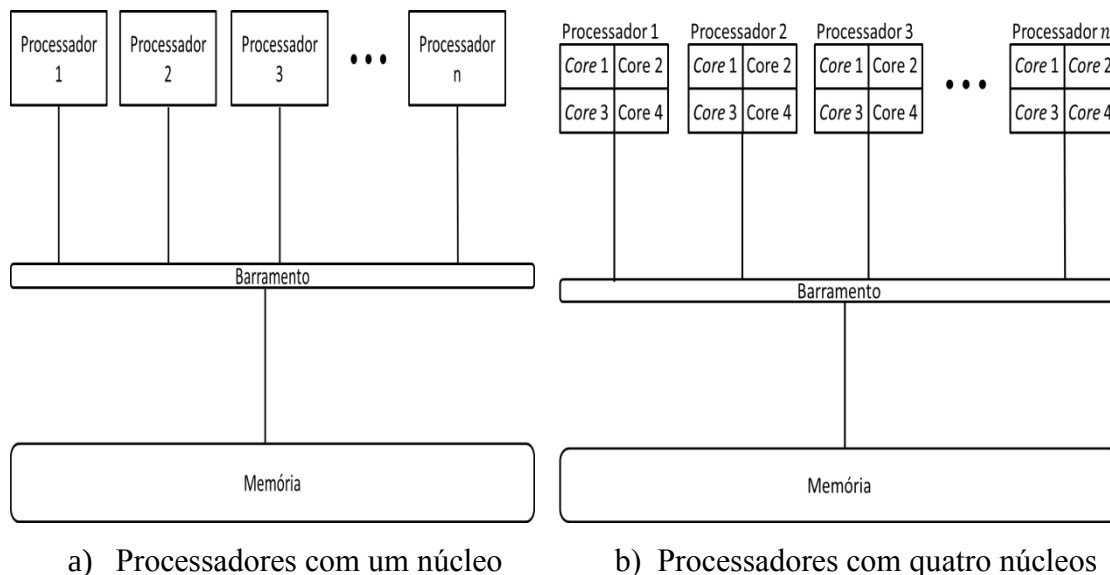
Figura 2.12: Representação de sistemas com memória compartilhada
