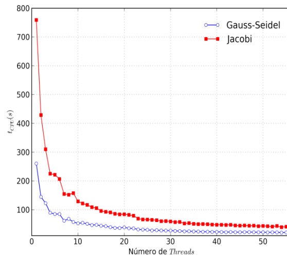
e) Tempo de CPU para N = 8193 \times 8193
