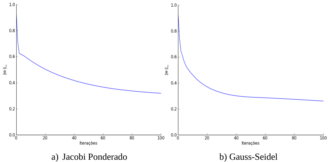
Figura 2.7: Métodos de Jacobi ponderado com \omega = 2/3 e Gauss-Seidel aplicados na estimativa inicial (v_1 + v_6 + v_{32})/3 ao longo de 100 iterações.
