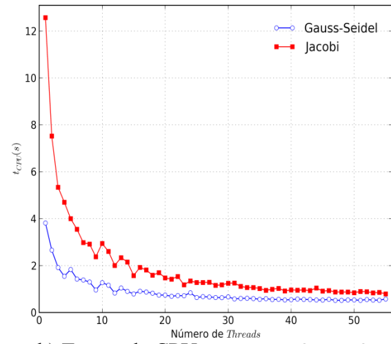
b) Tempo de CPU para N = 1025 \times 1025
