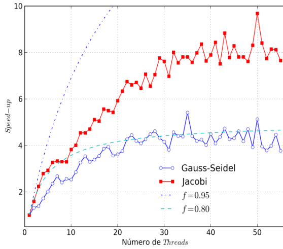
a) Speed-up para N = 513 \times 513
