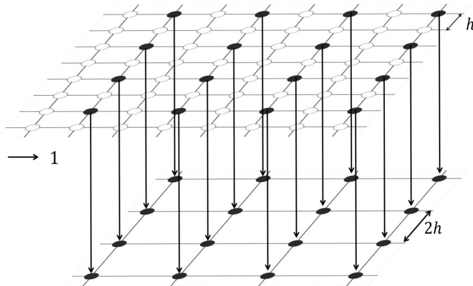
Figura 3.4: Restrição utilizando o operador de injeção.
