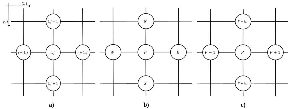
Figura 2.1: Nomenclatura dos vizinhos dos nós da malha bidimensional uniforme.
