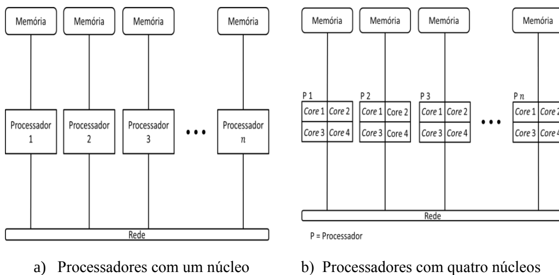
Figura 2.10: Representação de um cluster .
