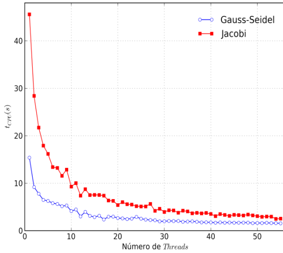
c) Tempo de CPU para N = 2049 \times 2049
