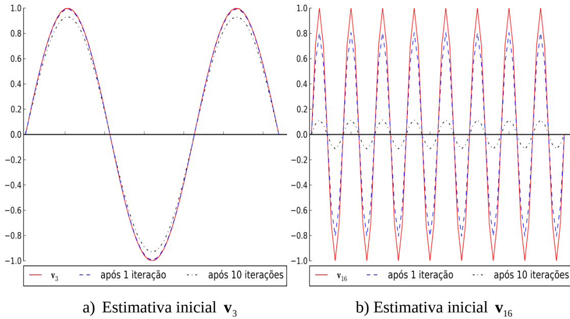
Figura 2.5: Método de Jacobi ponderado com \omega = 2/3 aplicado nas estimativas iniciais \mathbf{v}_3 e \mathbf{v}_{16} ao longo de 1 iteração e após 10 iterações (BRIGGS et al., 2000).
