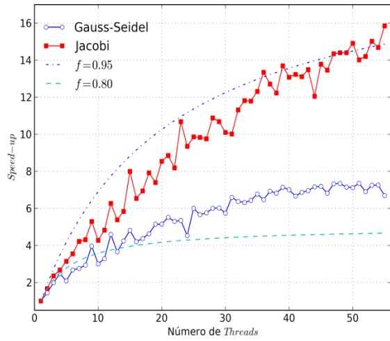
b) Speed-up para N = 1025 \times 1025
