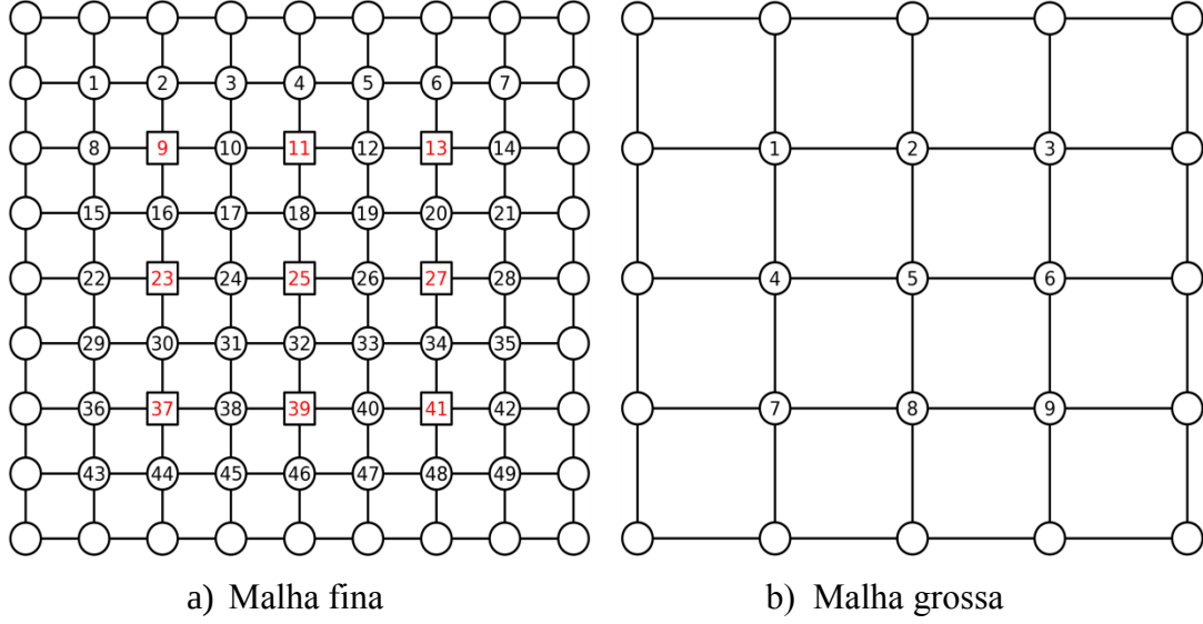
Figura 5.10: Relação entre nós efetivos de uma malha fina e malha grossa para razão de engrossamento r = 2 .
