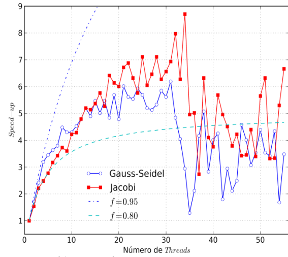
b) Speed-up para N = 257 \times 257
