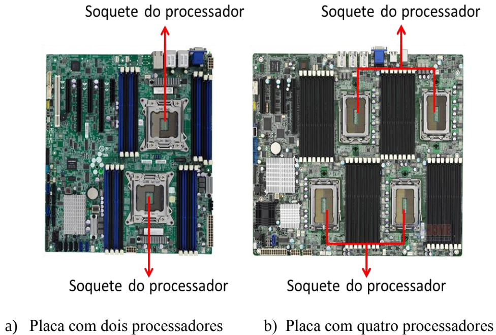
Figura 2.11: Placas mãe com mais de um soquete (onde são instalados os processadores).
