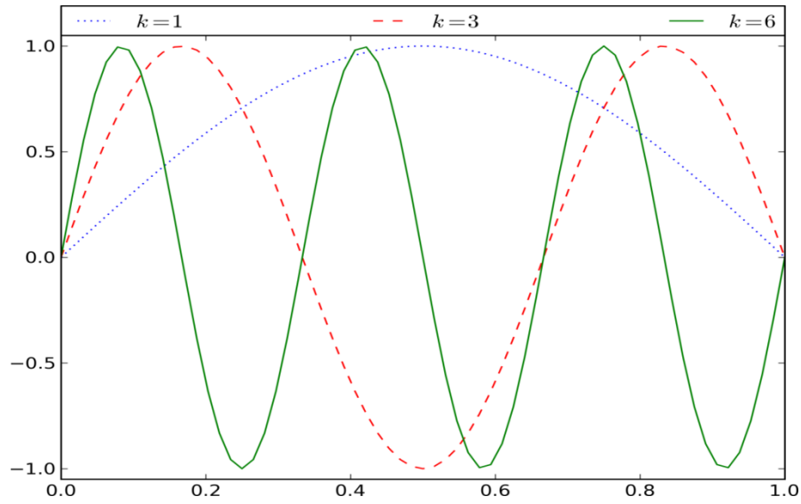
Figura 2.2: Modos de Fourier para k = 1, 3, 6 (BRIGGS et al., 2000).
