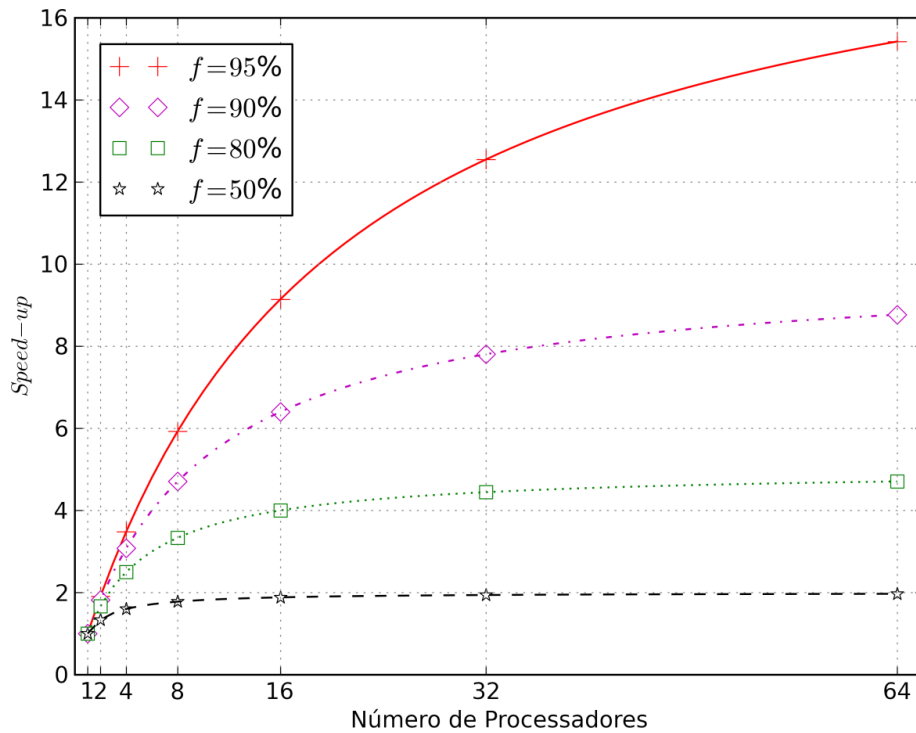
Figura 2.14: Limite superior de speed-up para programas com frações paralelas entre 50% a 95%.
