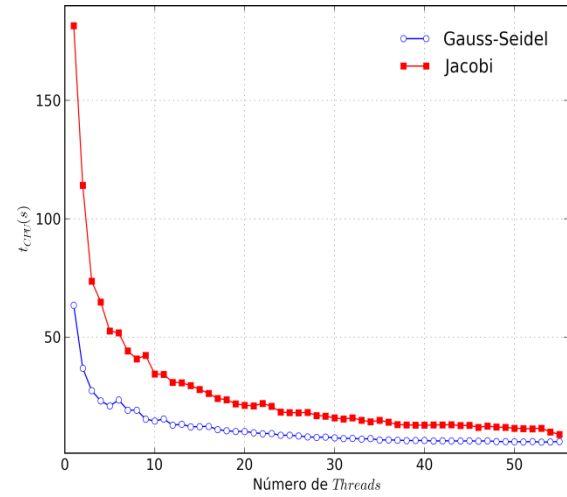
d) Tempo de CPU para N = 4097 \times 4097
