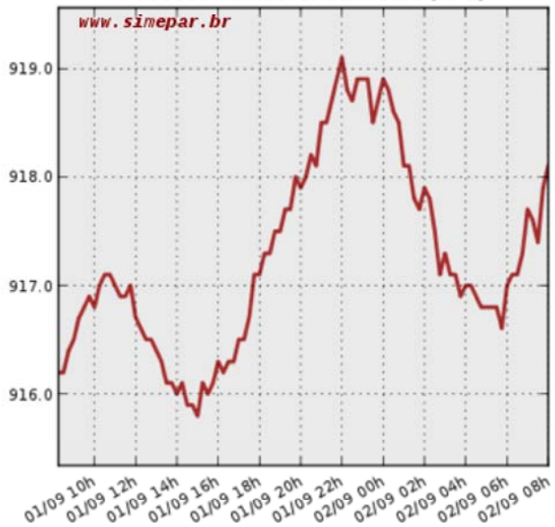
Pressão Atmosférica Média (hPa)
