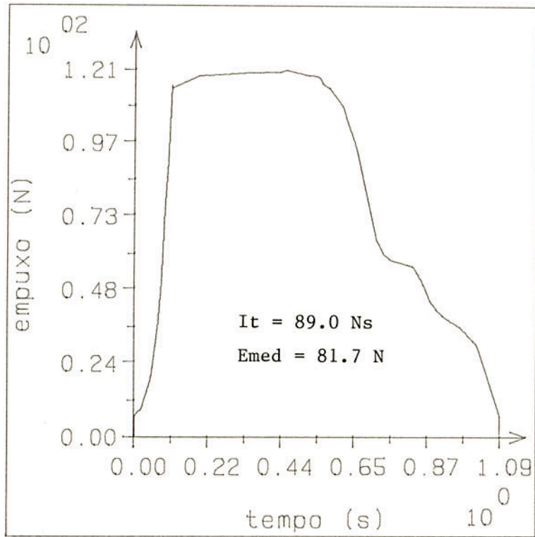
Figura 9. Curva de empuxo do TE-21.
