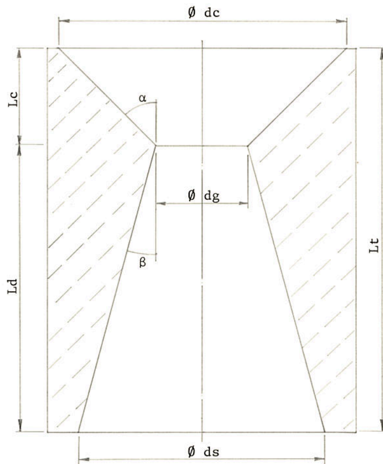
Figura 3. Parâmetros geométricos das tubeiras.
