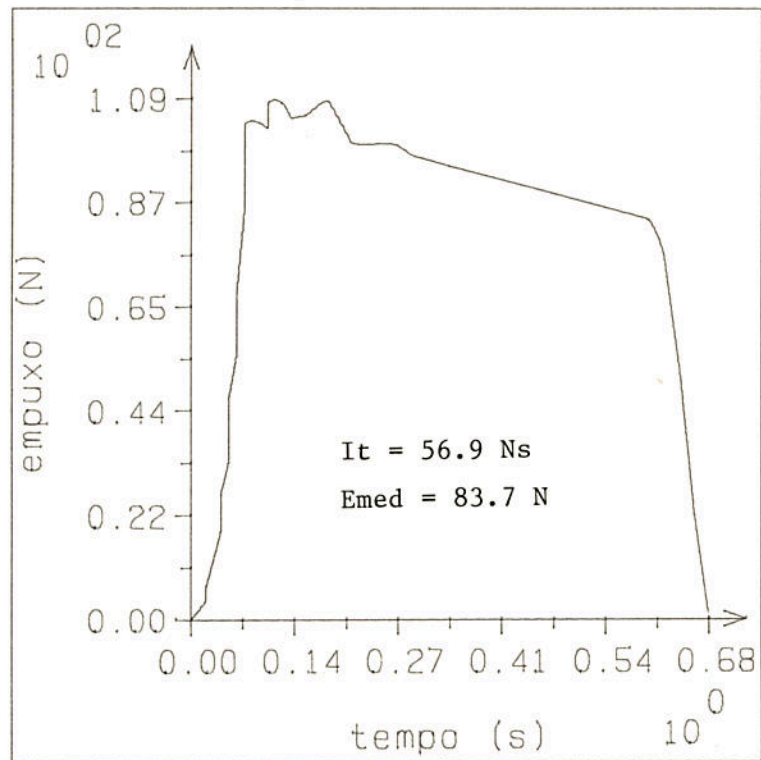
Figura 12. Curva de empuxo do TE-29.
