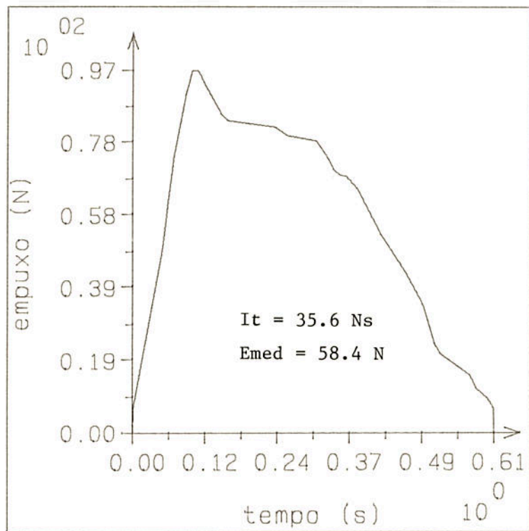
Figura 6. Curva de empuxo do TE-16.
