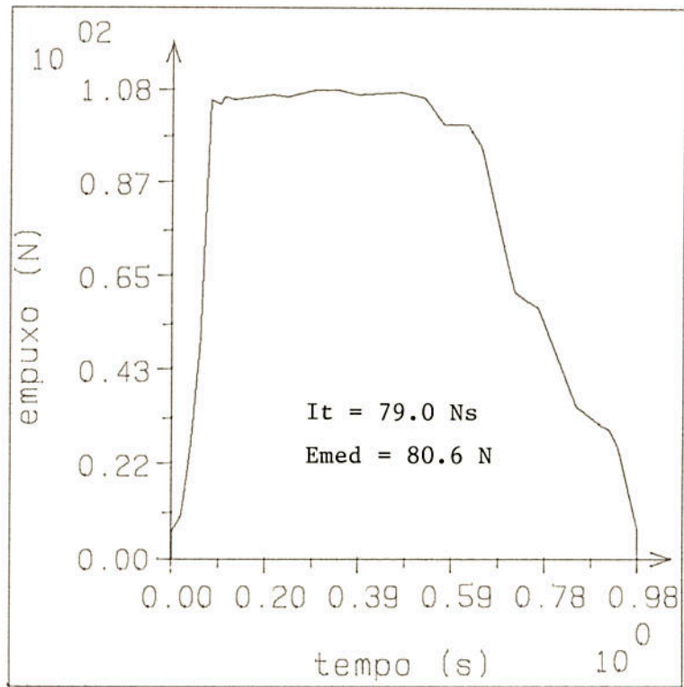
Figura 7. Curva de Empuxo do TE-19.
