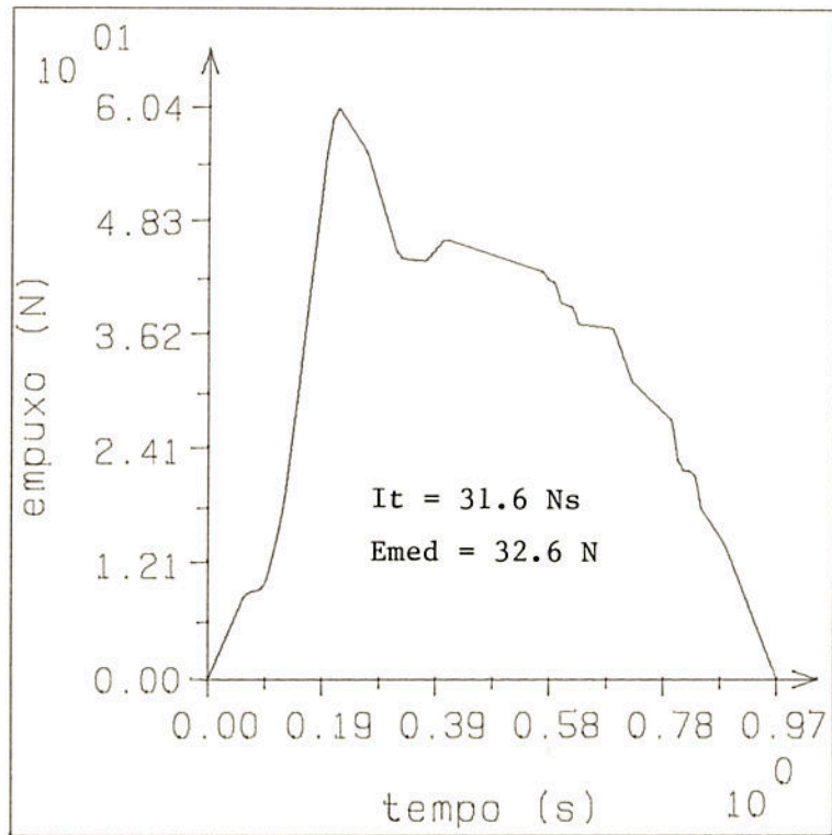
Figura 11. Curva de empuxo do TE-28.
