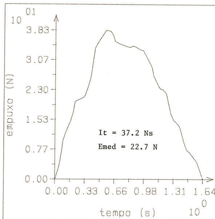
Figura 4. Curva de empuxo do TE-10.
