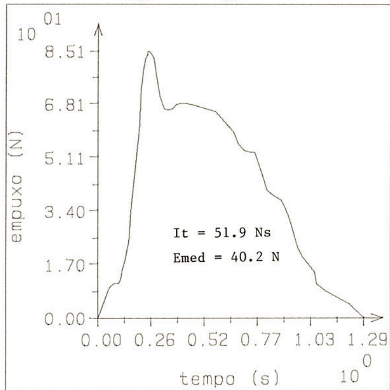
Figura 10. Curva de empuxo do TE-24.
