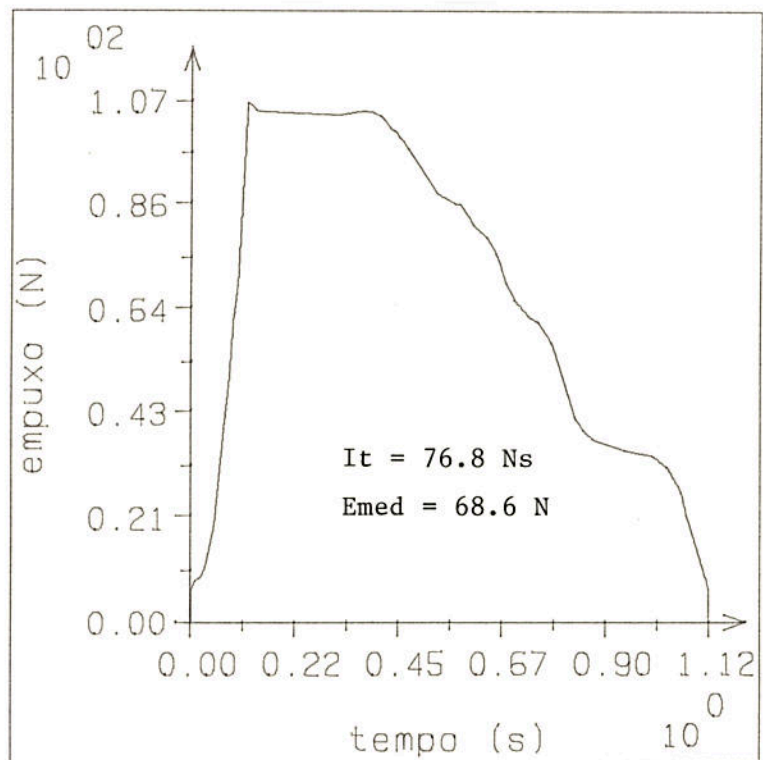
Figura 8. Curva de empuxo do TE-20.
