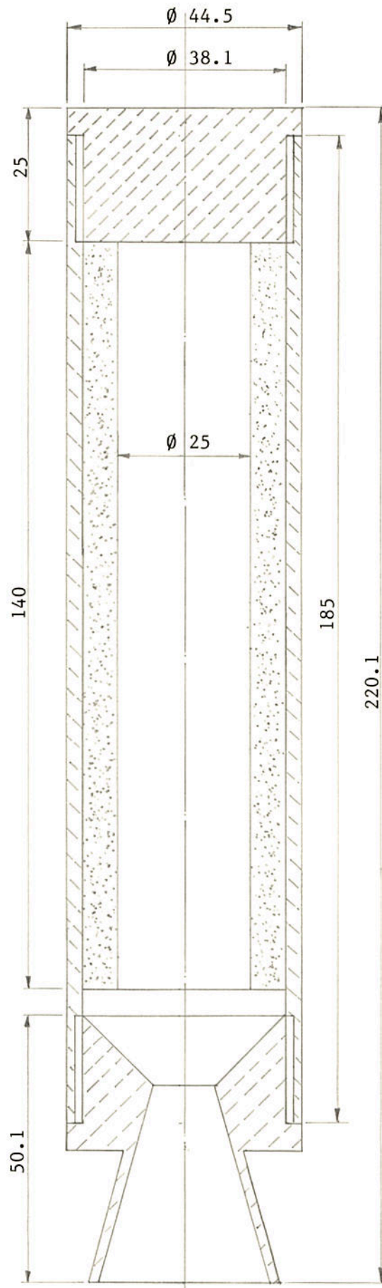
Figura 1. Motor-foguete Netuno-R.
