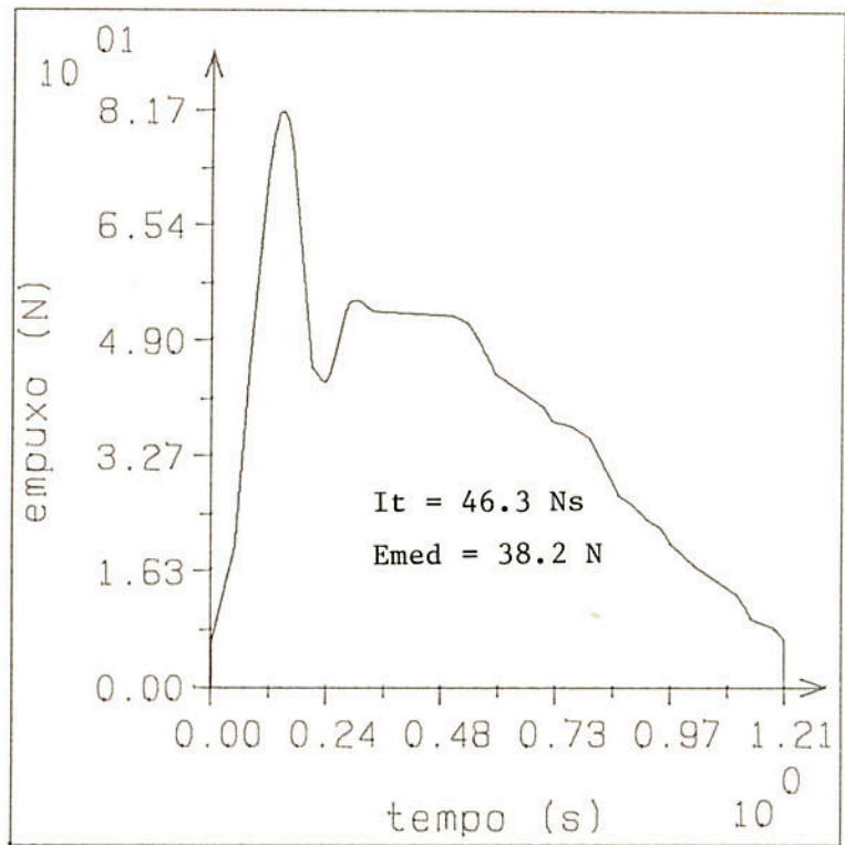
Figura 5. Curva de empuxo do TE-12.
