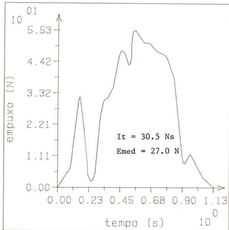
Figura 13. Curva de empuxo do TE-30.
