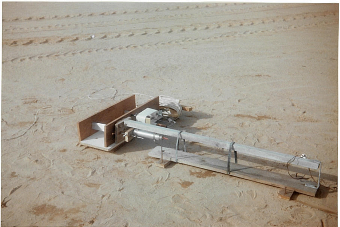
Foto 2. Banco estático BMB-1 com um minifoguete Netuno-R.
