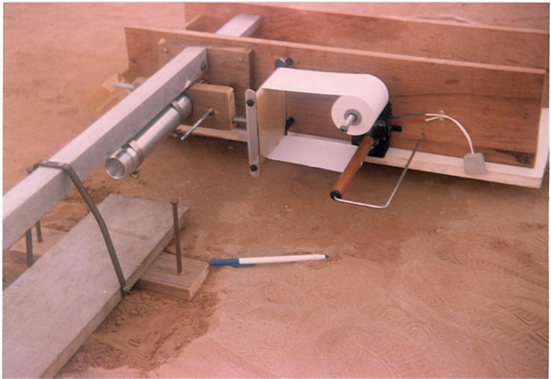
Foto 1. Detalhe do banco estático BMB-1 com um minifoguete Netuno-R.
