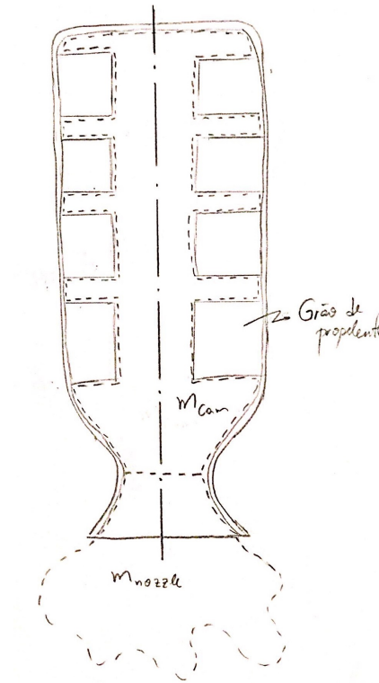
Figura 25 – Representação esquemática de vista em corte do motor, com indicação das massas do sistema
