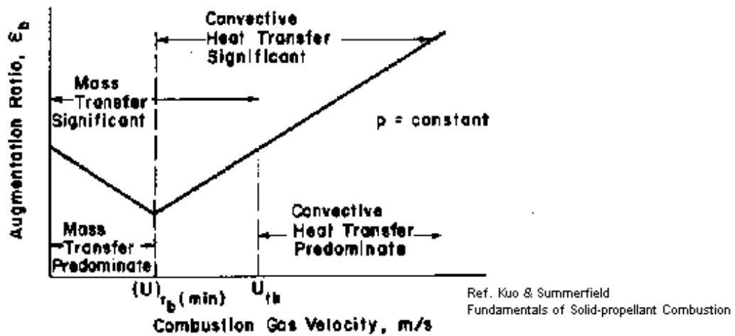
Figura 23 – Processo de transferência de calor que influencia a taxa de queima
