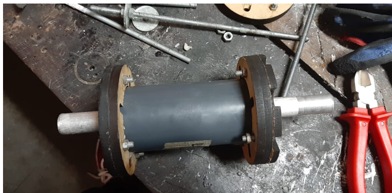
Figura 14 – Molde dos grãos
