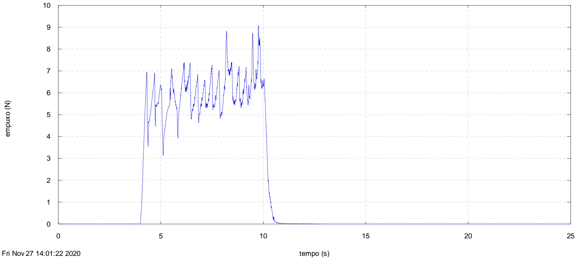
Motor LongBurn 3, TE 8 Jun 2013, Curva Empuxo 2.0.6.2
