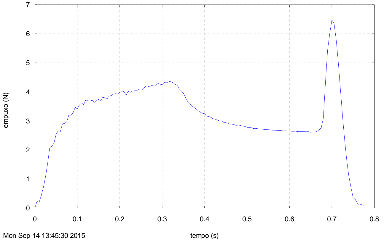
Motor BT311, TE 19 Ago 2015, Curva Empuxo 2.1
