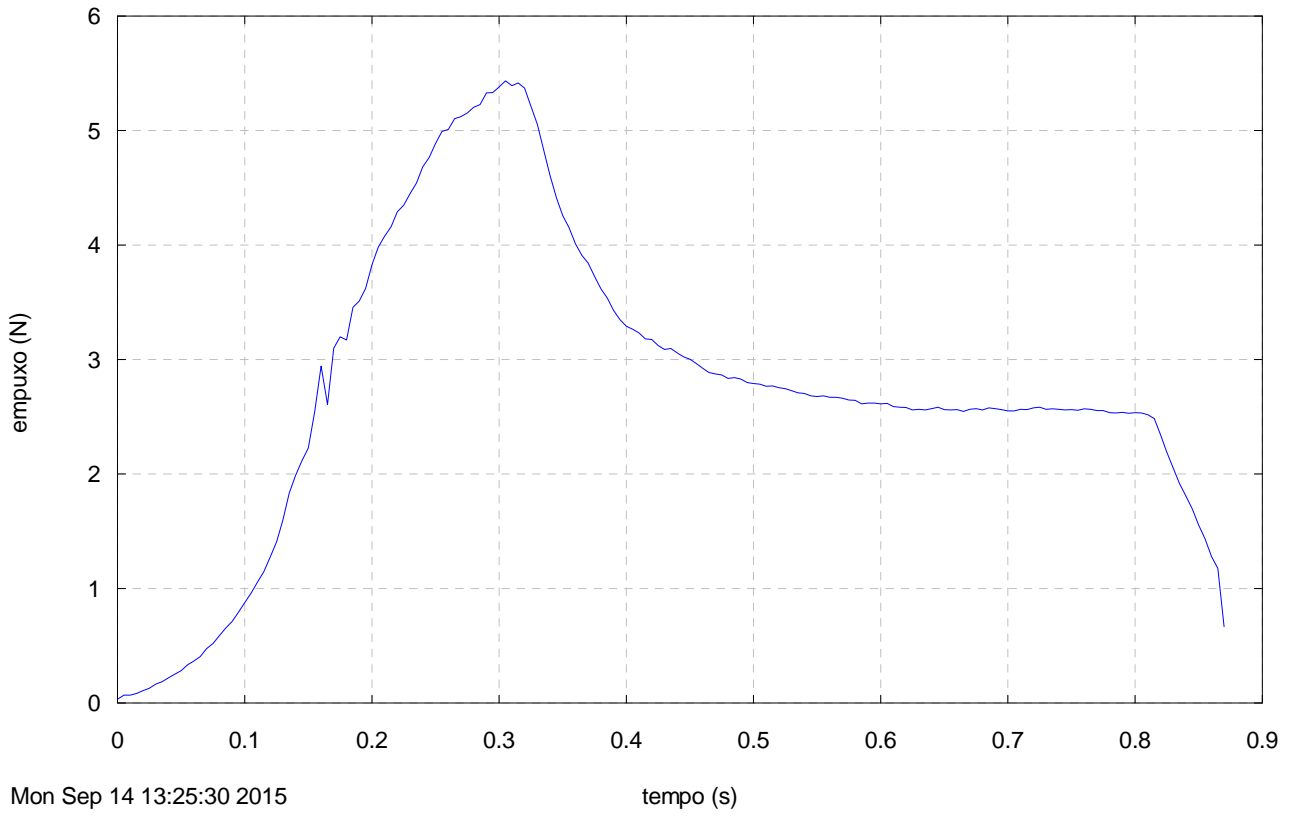
Motor U1, TE 19 Ago 2015, Curva Empuxo 2.1
