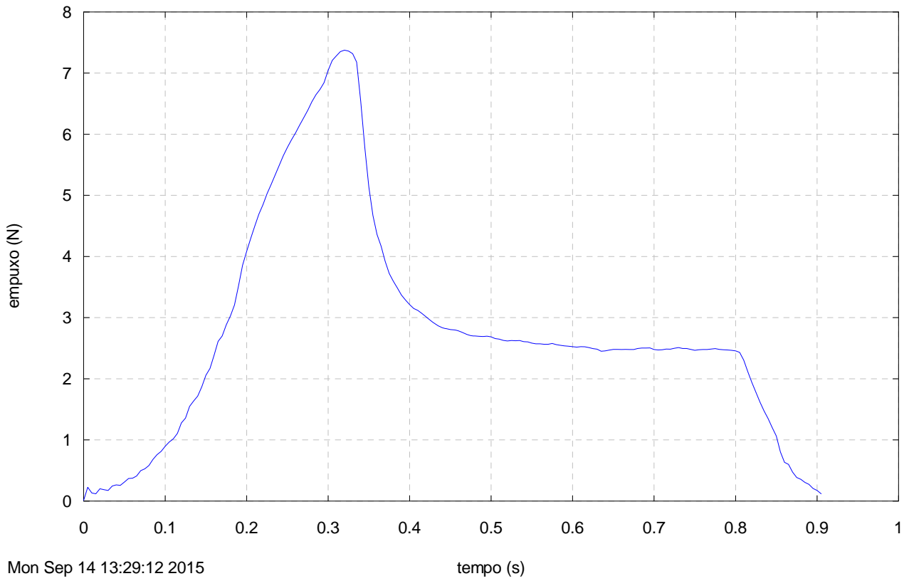
Motor U2, TE 19 Ago 2015, Curva Empuxo 2.1
