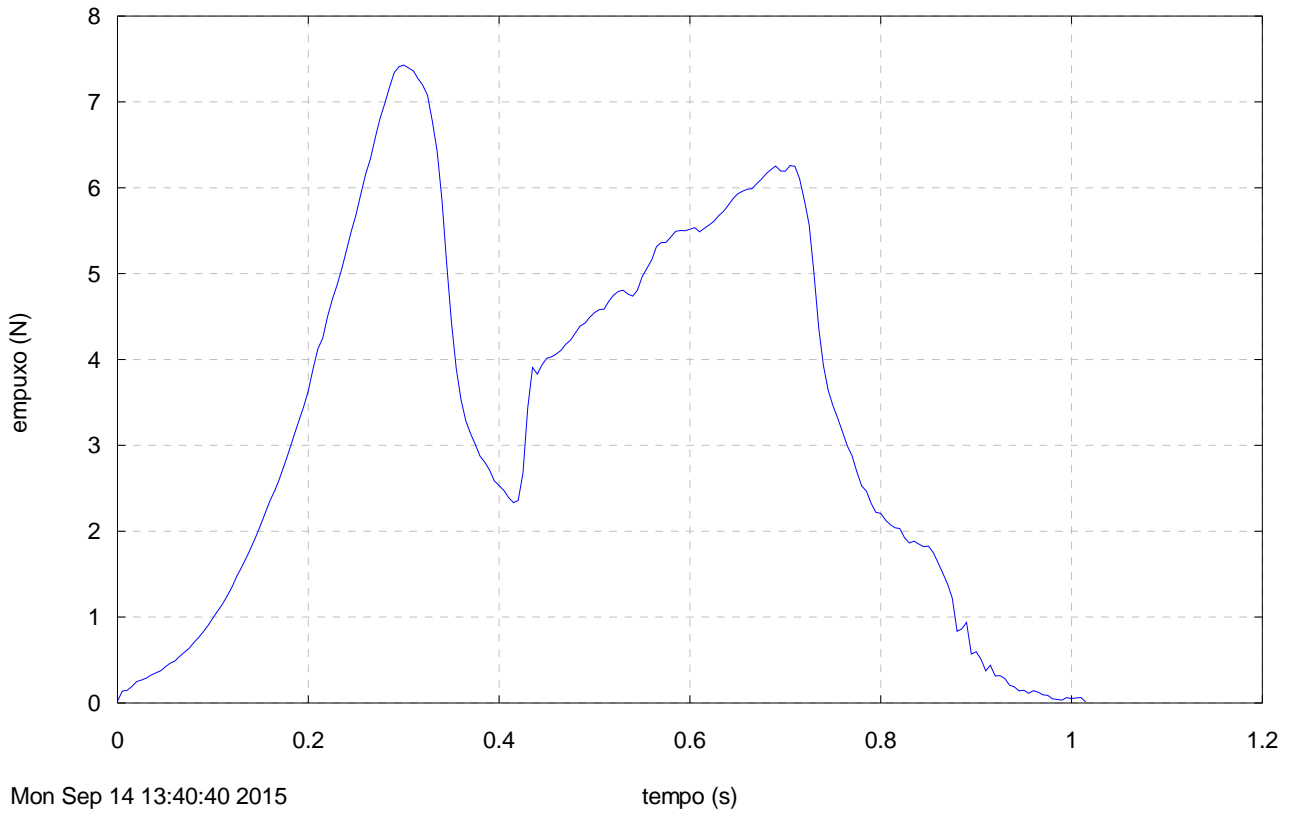
Motor U5, TE 19 Ago 2015, Curva Empuxo 2.1
