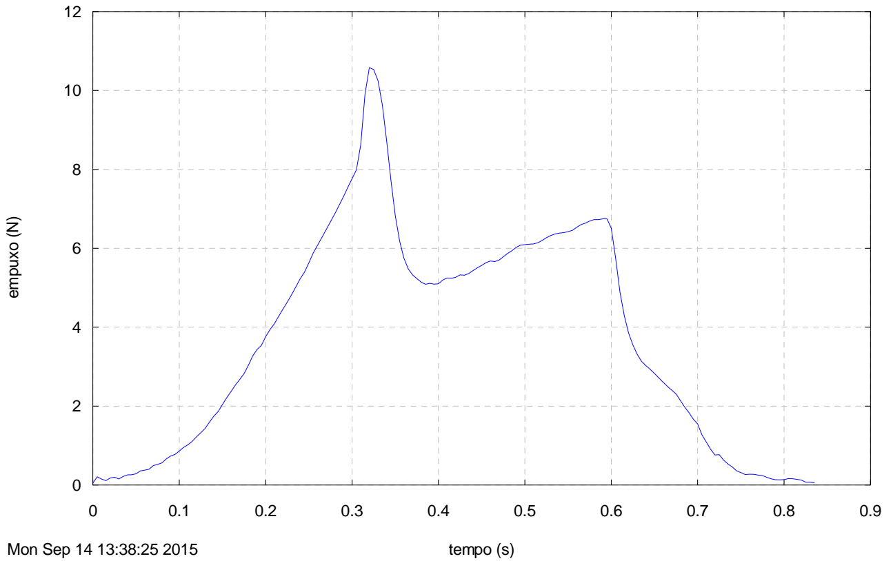
Motor U4, TE 19 Ago 2015, Curva Empuxo 2.1
