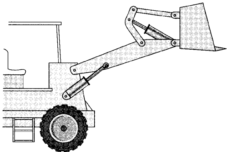
Pá Carregadeira
