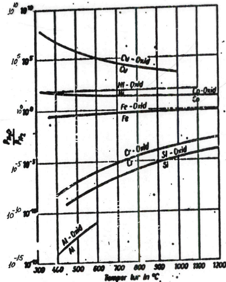
Bild 0.36. Gleichgewichtskurven für die Oxidbildung (nach [0.20])
