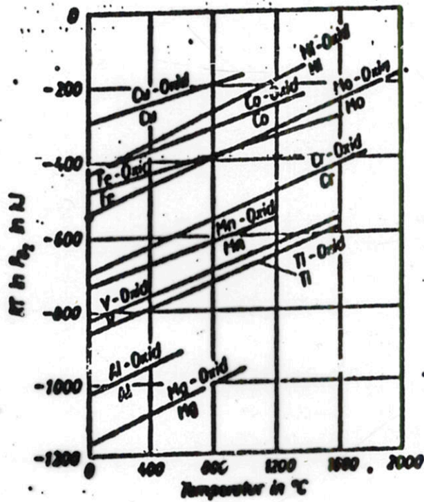
Bild 0.35. Änderung der freien Enthalpie \Delta G der Oxidbildung von Metallen (nach [6.20])
