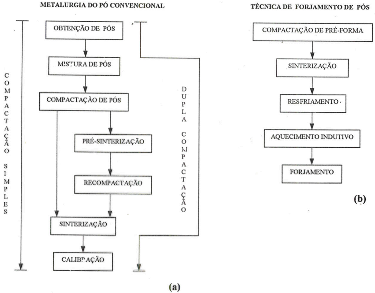
Figura 2.2- Representação esquemática das principais etapas do processo de fabricação de componentes mecânicos ferrosos via MP: pela MPC (a) e pela TFP (b).
