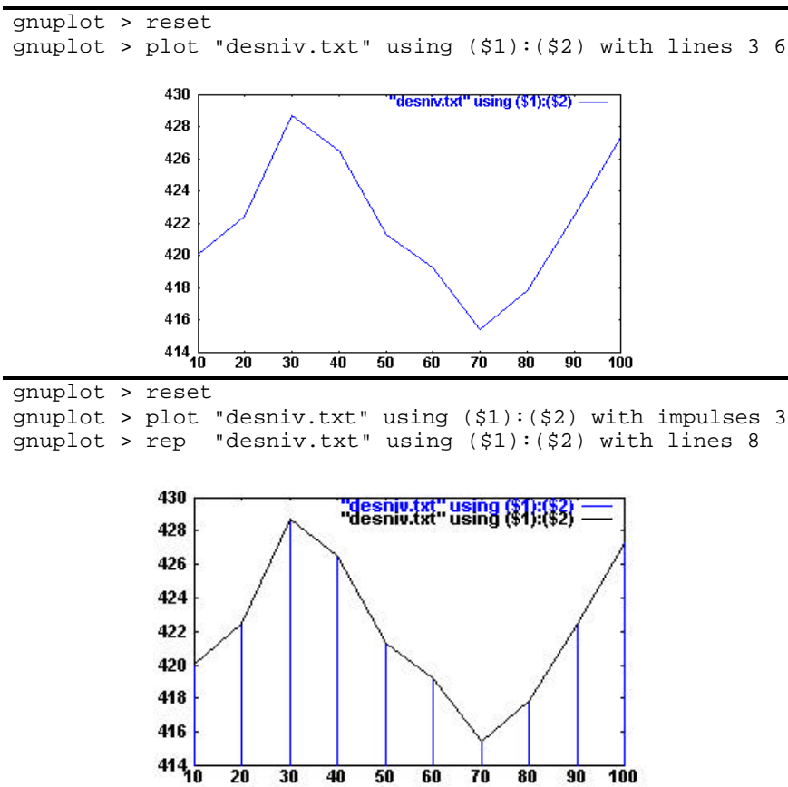
Figura 5.3 – Visualização de dados lidos em arquivo, com mudança de atributos.
